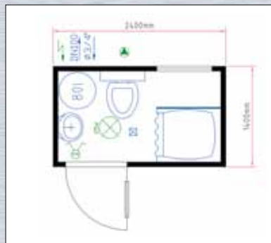
Grundriss 8' WC-Dusch- Container
