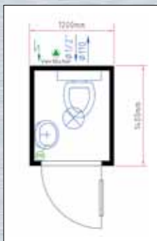
Grundriss 5' WC-Container
