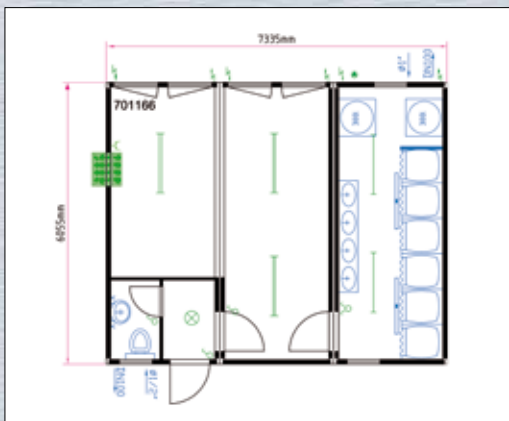
Grundriss-Beispiel 3er-Anlage
