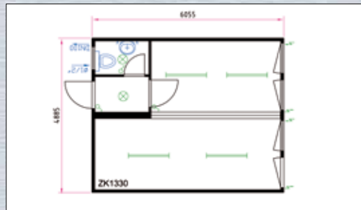
Grundriss-Beispiel 2er-Anlage
